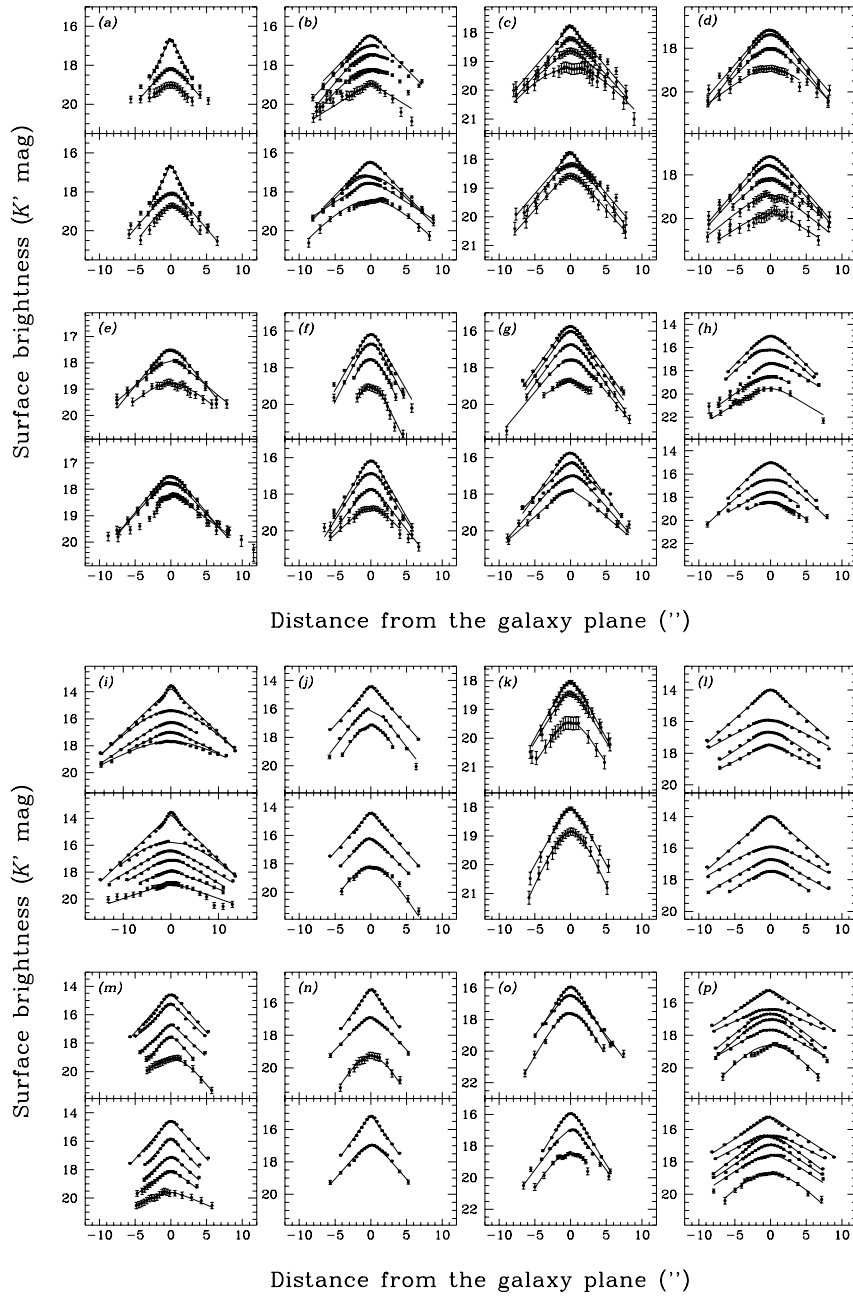
Fig. 5a–x. Vertical K -band luminosity profiles for the sample galaxies: a ESO026G-06; b ESO041G-09; c ESO141G-27; d ESO142G-24; e ESO157G-18; f ESO201G-22; g ESO263G-15; h ESO286G-18; i ESO311G-12; j ESO315G-20; k ESO340G-09; l ESO358G-29; m ESO383G-05; n ESO416G-25; o ESO435G-14; p ESO435G-25.
